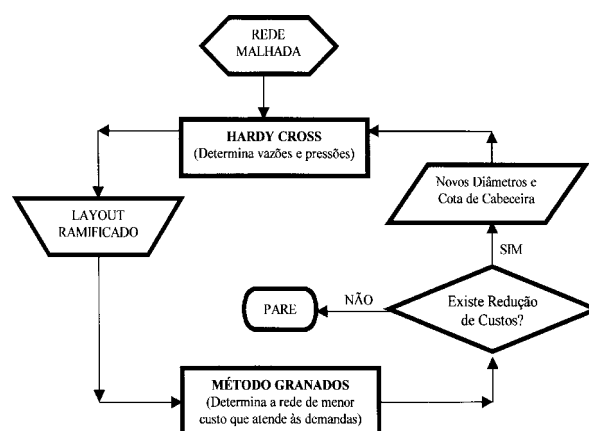
Figura 1. Algoritmo da junção do método GRANADOS com o método HARDY CROSS.
