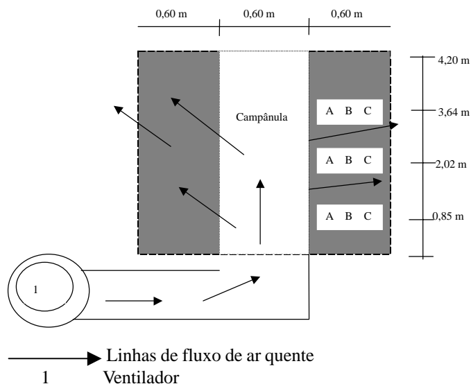
Figura 1. Corte transversal do secador mostrando os pontos de amostragem
