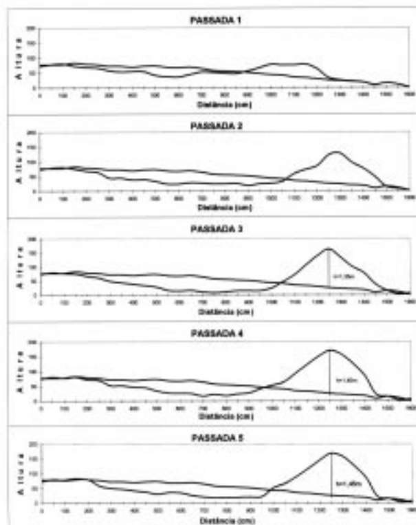
Figura 3. Seqüência das seções transversais do terraço a cada passada da máquina
