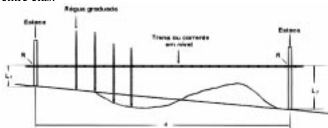
Figura 1. Esquema de levantamento do perfil do terraço
