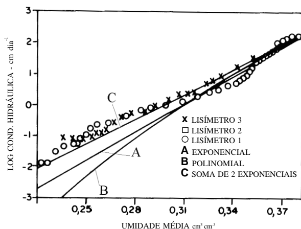
Figura 5. Curvas de ajustamento para relação entre a condutividade hidráulica e teor de umidade do solo a 25 cm de profundidade, para diferentes lisímetros. (A) Exponencial, (B) Polinomial e (C) Soma de duas exponenciais
