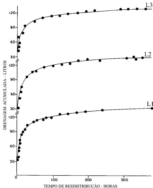
Figura 1. Drenagem acumulada em função do tempo para diferentes lisímetros (L)
