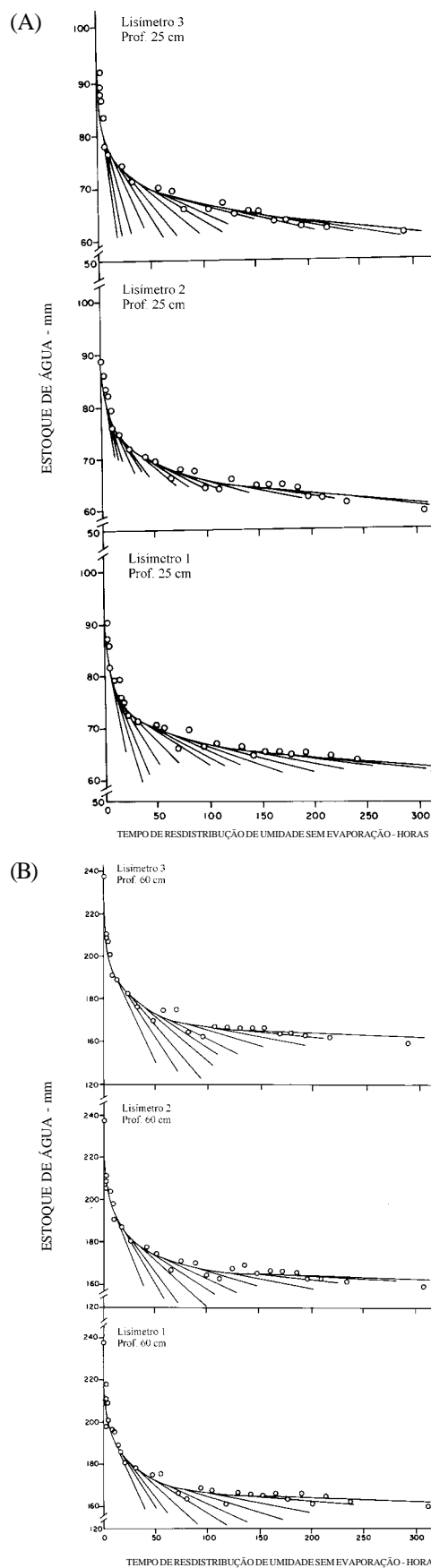
Figura 2. Curvas de armazenamento de água referentes à camada de (A) 25 e (B) 60 cm do solo, durante a drenagem interna, com tangente em pontos específicos do tempo para os três lisímetros utilizados
