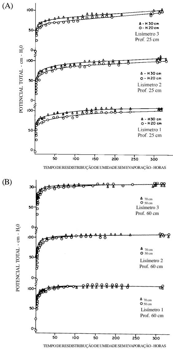
Figura 3. Evolução do potencial total de água no solo (A) 20/30 cm e (B) 50/70 cm de profundidade, durante a drenagem interna, para diferentes lisímetros
