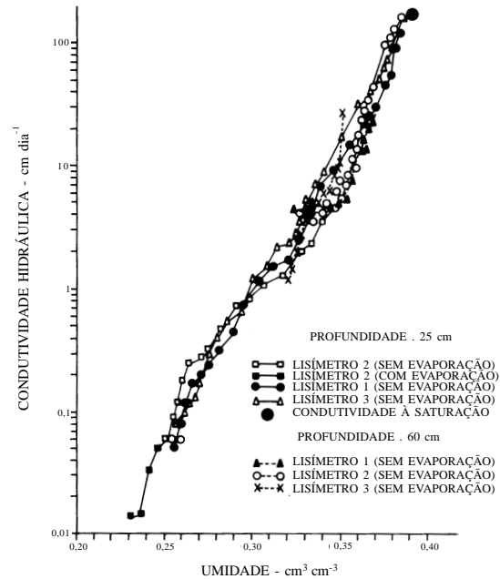
Figura 4. Curvas de condutividade hidráulica do solo em função da umidade média a 25 e 60 cm de profundidade, para diferentes lisímetros
