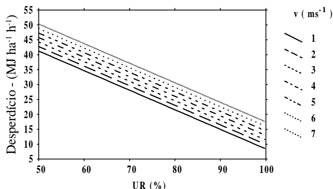
Figura 1. Estimativa do desperdiço de energia em função da umidade relativa do ar (UR) para diferentes velocidades do vento (v), radiação solar de 520 Wm -2 e pressão de serviço do aspersor de 686 kPa
