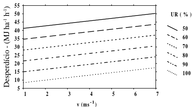
Figura 2. Estimativa do desperdiço de energia em função da velocidade do vento (v) para diferentes umidades relativas (UR), radiação solar de 520 Wm -2 e pressão de serviço do aspersor de 686 kPa
