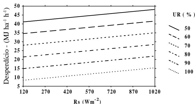
Figura 5. Estimativa do desperdício de energia em função da radiação solar (Rs) para diferentes umidades relativas (UR), velocidade do vento de 3 m s -1 e pressão de serviço do aspersor de 686 kPa
