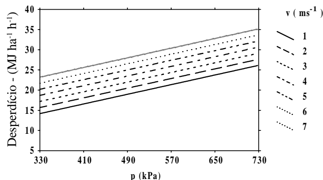
Figura 3. Estimativa do desperdiço de energia em função da pressão de serviço do aspersor (p) para diferentes velocidades do vento (v), radiação solar de 520 W m -2 e UR de 75%
